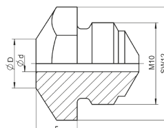
Modelo especial 17/.....Boquillas Plástico
