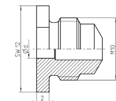
Modelo especial 17/.....Boquillas Plástico
