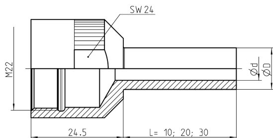
Modelo prolongada FireBird®
