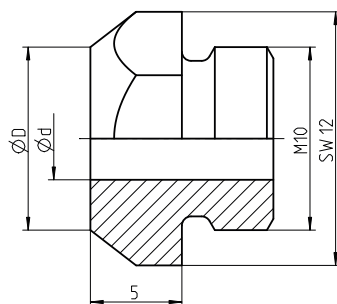
Modelo estándar 17/.....Boquillas
