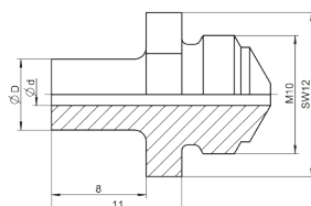
Modelo especial 17/.....Boquillas BT
