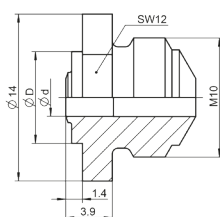
Modelo especial 17/.....Boquillas MB
