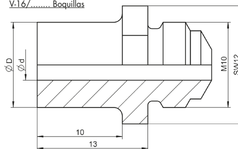
Versión prolongada (10 mm) V-16/..... Boquillas
