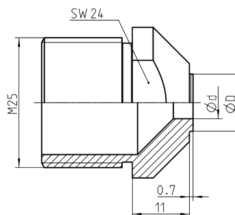
Modelo estándar FireBird® Pro/FireFox®
