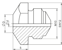
Modelo estándar 17/.....Boquillas
