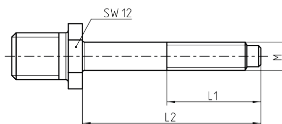
Modelo estándar FireBird® Pro/FireFox®
