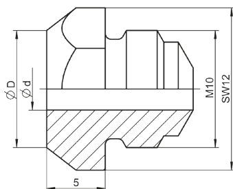
Versión estándar 16/..... Boquillas
