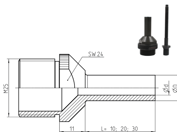
Modelo prolongada FireBird® Pro/FireFox®
