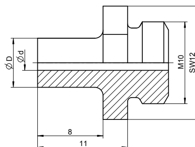
Modelo prolongado (8 mm) V-17/.....Boquillas
