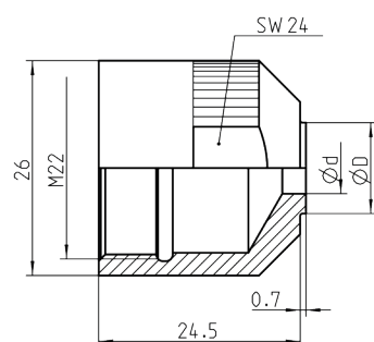
Modelo estándar FireBird®
